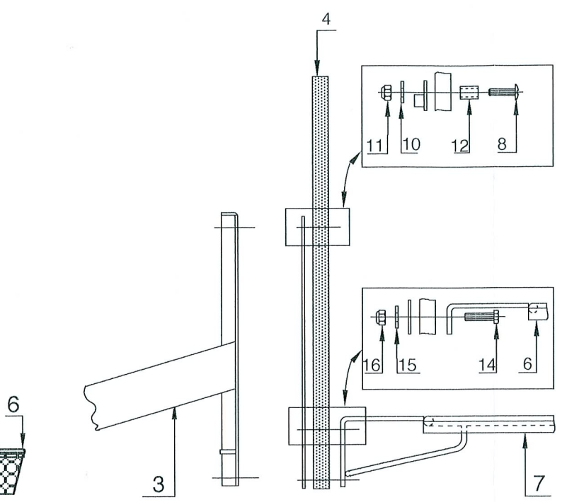
Montage du cercle et du panneau fibreglass
