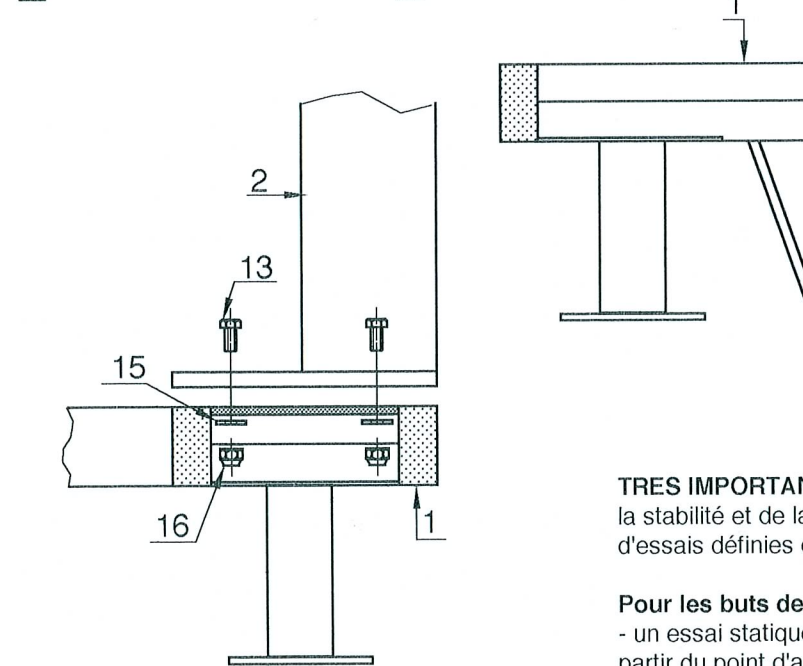
Montage du pied sur le chassis
