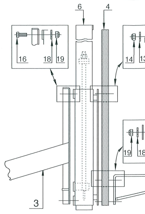
Montage du système de réglage et du panneau fibreglas
