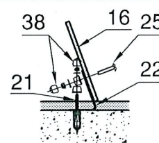
Fixation de l'équerre de scellement du mur d'escalade.
