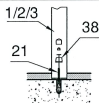
Fixation des pieds du jeu.
