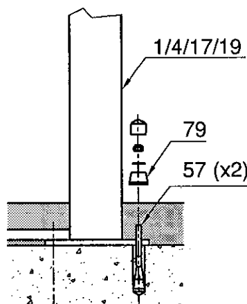
Fixation des pieds des tours A et B.
