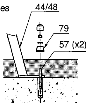
Fixation des pieds du mur d'escalade et des pieds intermédiaires de la glissière ht. 2,45m.
