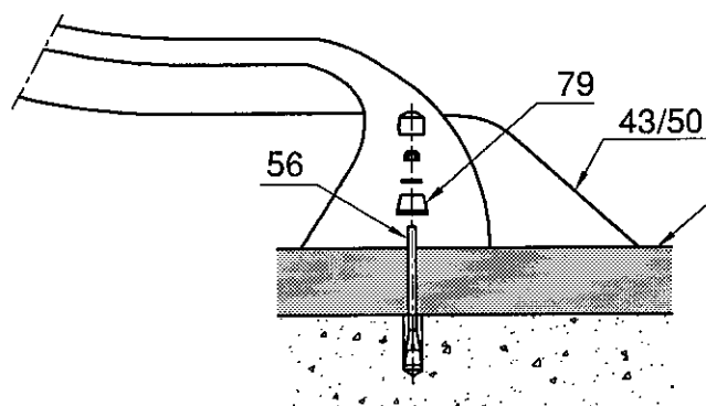
Fixation des glissières.
