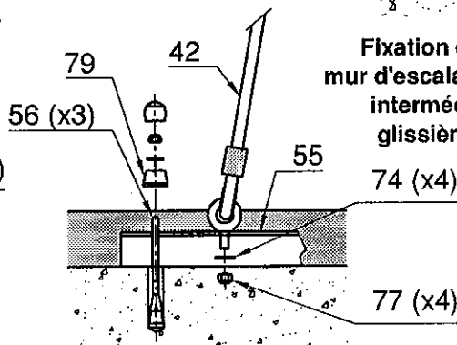
Fixation du filet à grimper.
