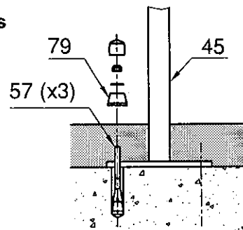
Fixation du mât de pompiers.
