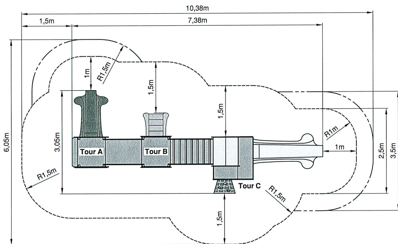
Position du jeu par rapport à l'espace minimal libre et à la surface d'impact.
