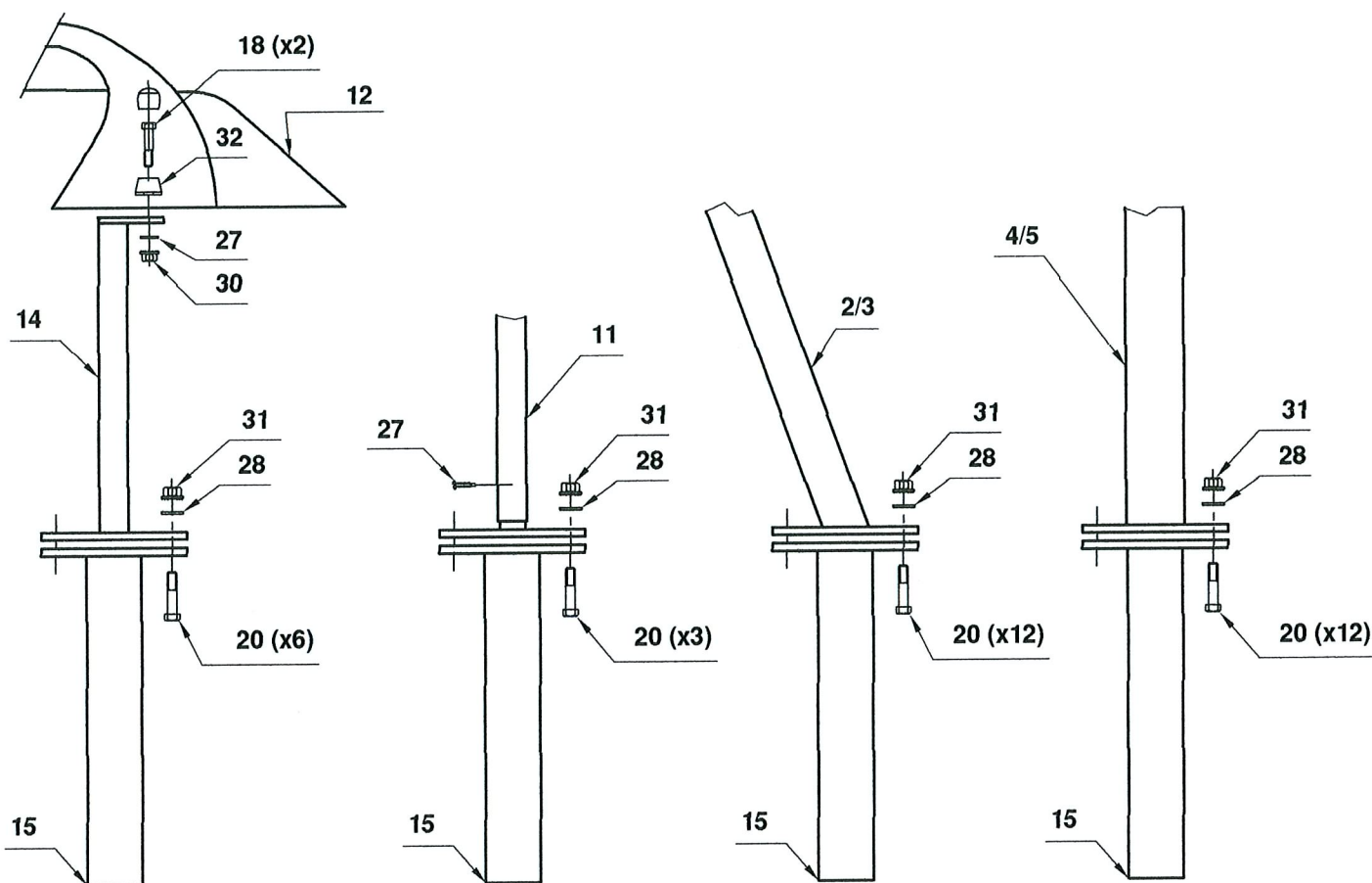
Montage pieds de scellement des tours.
