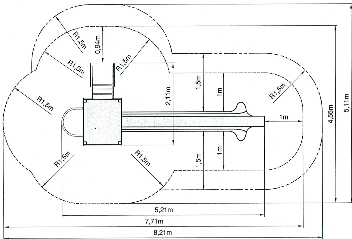
Position du jeu par rapport à l'espace minimal libre et à la surface d'impact
