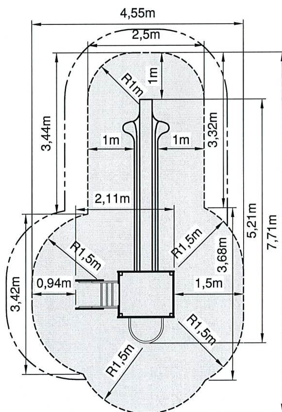
Position du jeu sur sol coulé.
