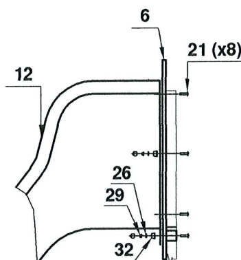
Assemblage de la glissière sur la tour
