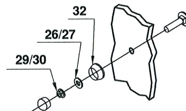
Montage identique pour toutes les vis sauf indication contraire.
