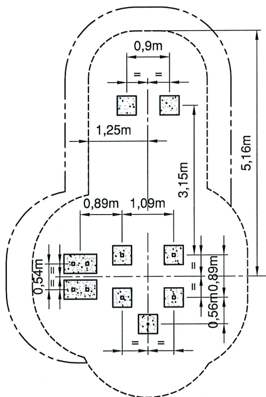
Position des massifs béton éventuel sur sol souple (dalles ou sol coulé)
