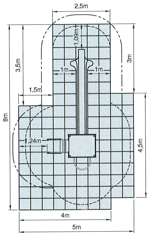
Position du jeu sur dalles souples en décaissé.
