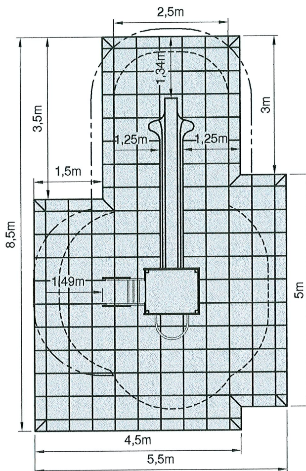
Position du jeu sur dalles souples en pose directe.
