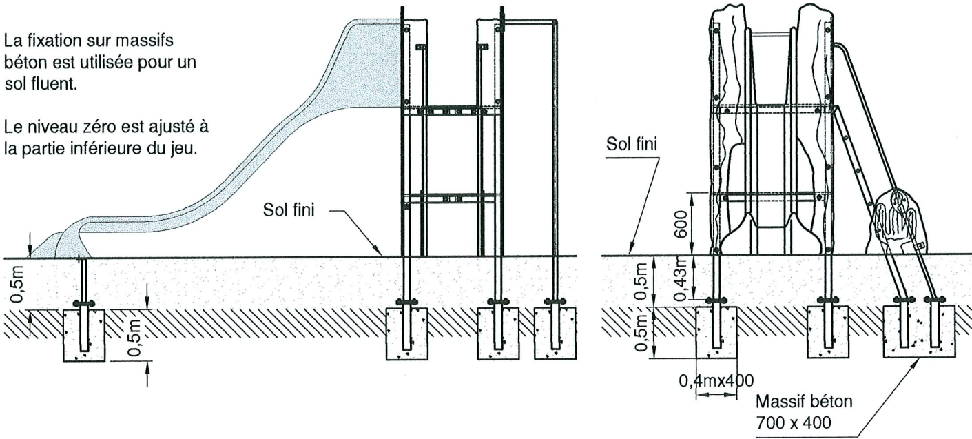
Position du jeu sur sol fluant (sable, gravier, écorces ou copeaux)
