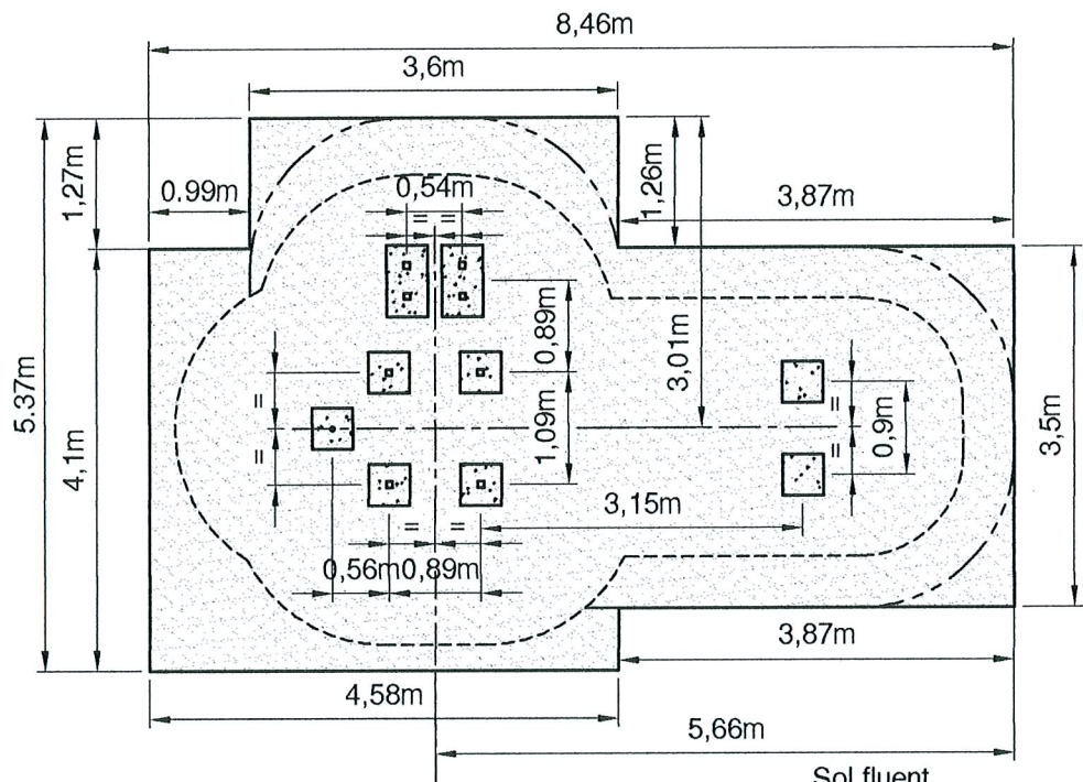
Position du jeu sur sol fluant (sable, gravier, écorces ou copeaux)
