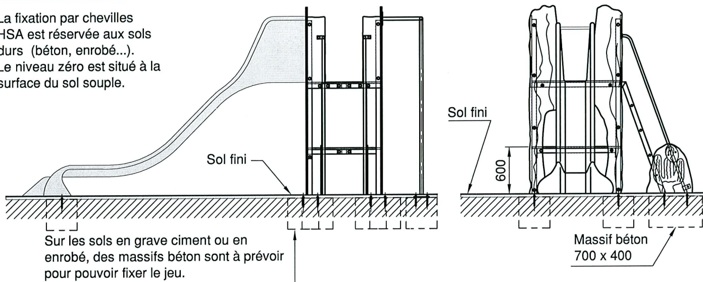
Position du jeu sur sol coulé.
