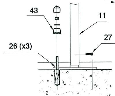
Fixation du mât de pompier.
