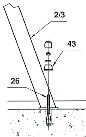
Fixation des pieds de l'échelle et de la rambarde.
