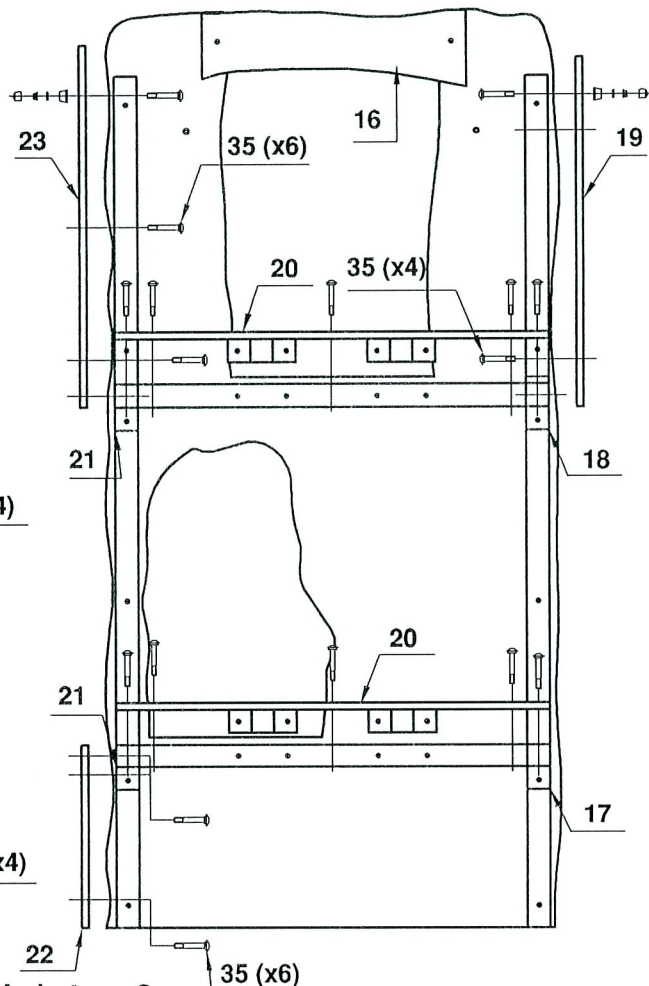
Assemblage de la tour 2
