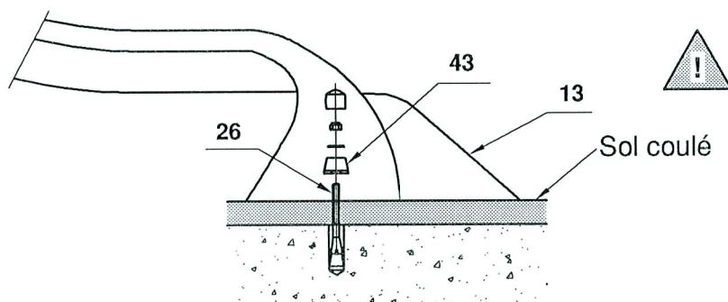
Fixation des glissières.
