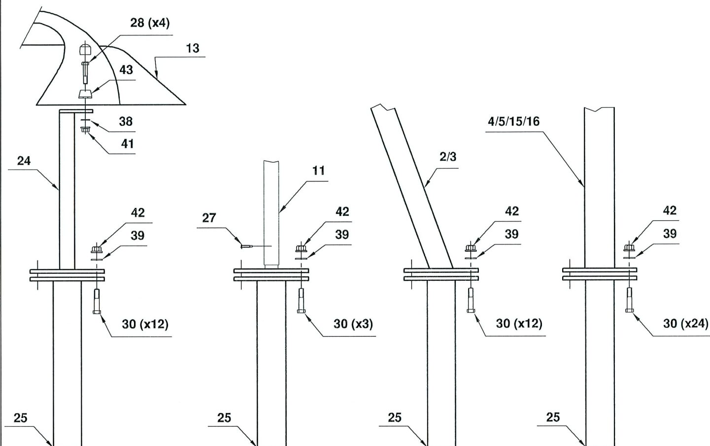
Montage pieds de scellement glissières.
