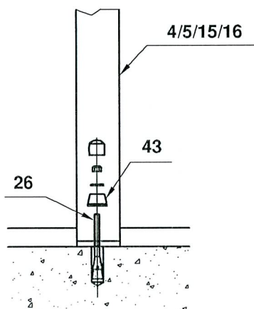
Fixation des pieds des tours 1 et 2.
