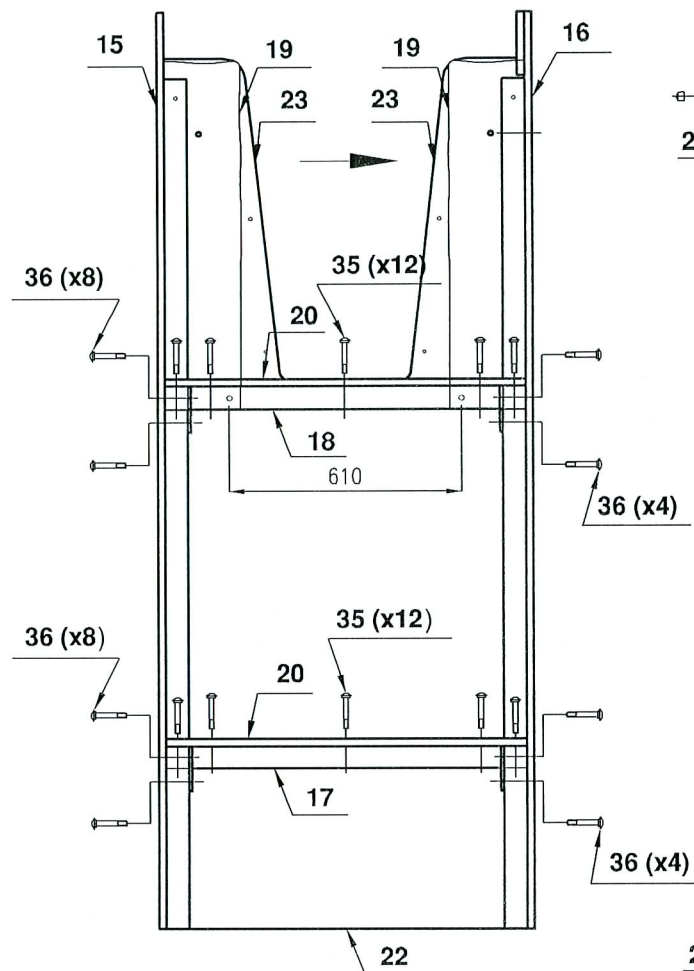
Assemblage de la tour 2
