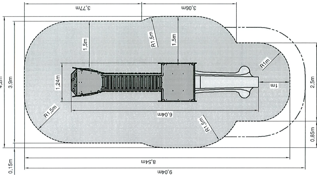
Position du jeu sur sol coulé.
