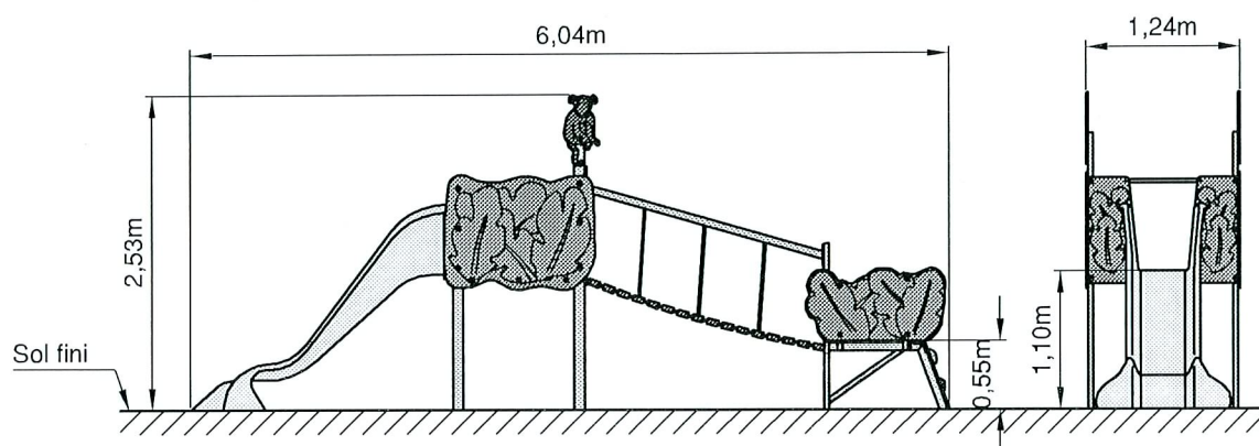
Position du jeu par rapport à l'espace minimal libre et à la surface d'impact.
