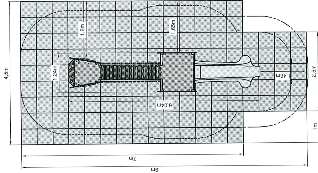
Position du jeu sur dalles souples en décaissé.
